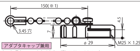
レセプタクルキャップ: NCS-25-RCa
