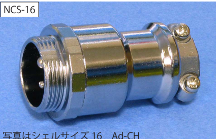
写真はシェルサイズ 16 Ad-CH
