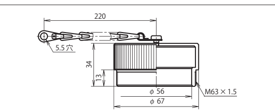
プラグキャップ：NCS-60-PCa
