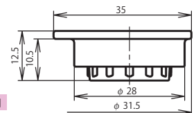
レセプタクルキャップ：NR-24-RCa・1
