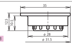
レセプタクルキャップ：NR-24-RCa・1
