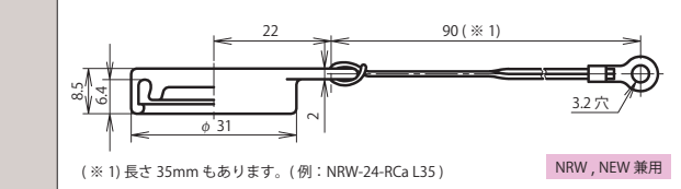
レセプタクルゴムキャップ: NRW-24-RCa
