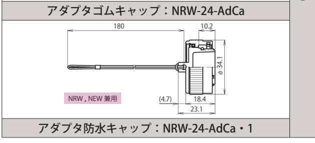
アダプタゴムキャップ: NRW-24-AdCa
