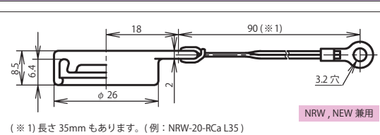
レセプタクルゴムキャップ: NRW-20-RCa
