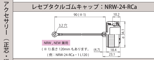
レセプタクル防水キャップ: NRW-24-RCa・1
