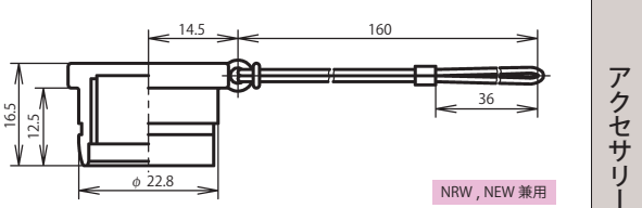
プラグ防水キャップ: NRW-20-PCa・1
