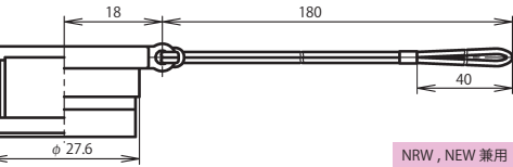
プラグ防水キャップ: NRW-24-PCa・1
