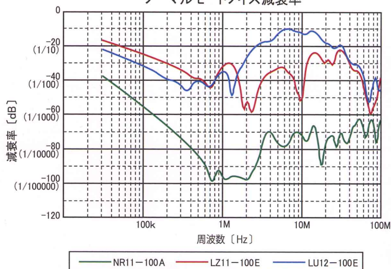
ノーマルモードノイズ減衰率
