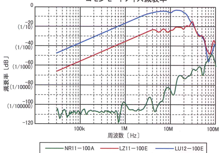
コモンモードノイズ減衰率
